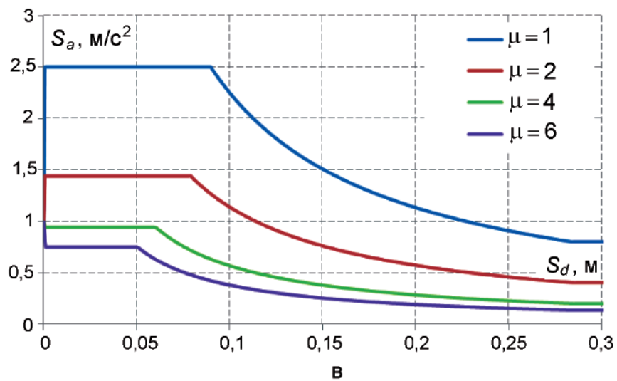
Рисунок Д.2 – Графіки " S_a - S_d " за сейсмічних впливів інтенсивністю 7 балів і різних коефіцієнтах податливості \mu будівлі (споруди)
